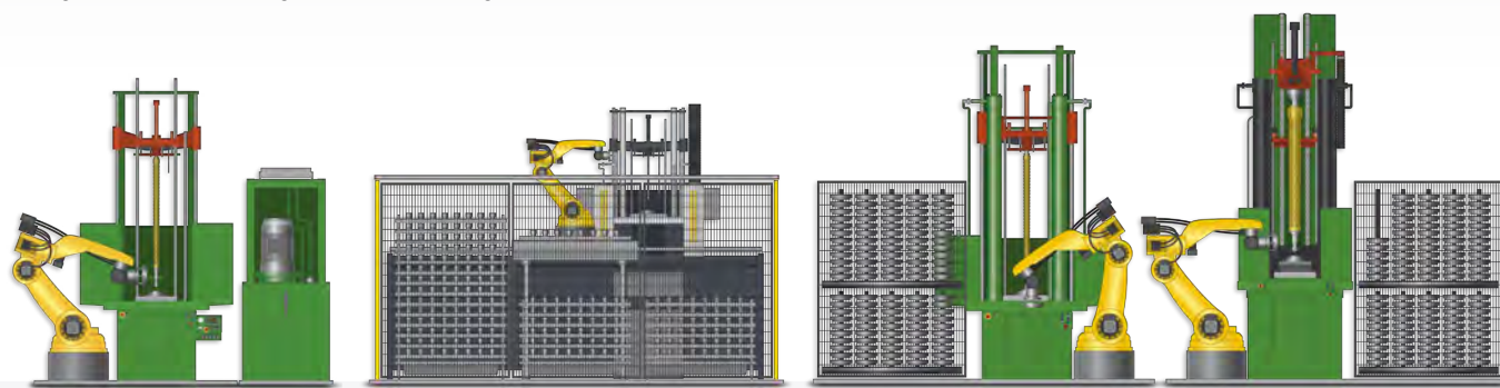
VRV Brocciatrice Automatizzata 15 Ton corsa 1200 mm con guida broccia
