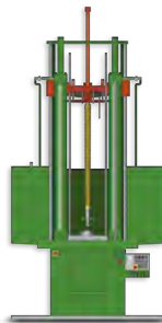
VRV Brocciatrice 25 Ton corsa 1800 mm con guida broccia
